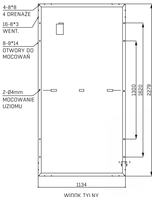
WIDOK TYLNY
